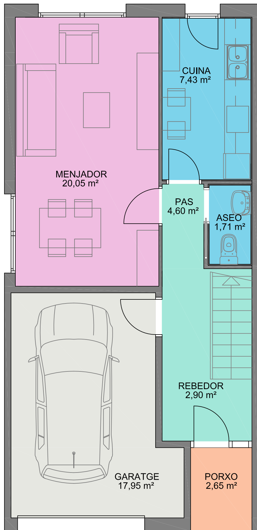
PLANTA BAIXA TIPUS CANTONERA
